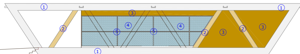
Alçado longitudinal
