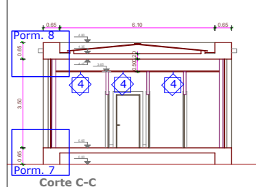
Corte C-C
